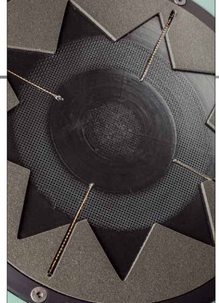
Der „Stern“ bildet den optisch unverwechselbaren Dämpfer auf der Membran des BiegeWellenwandlers
